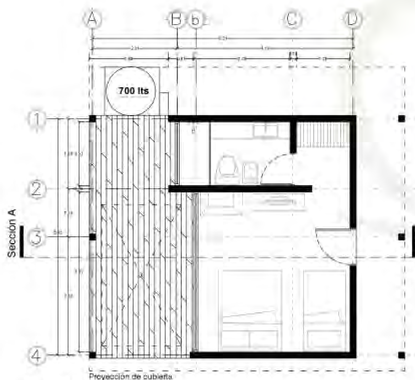
PLANTA BAJA
